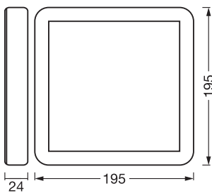
ORBIS QUICKFIX195X19516WCLICKD830
