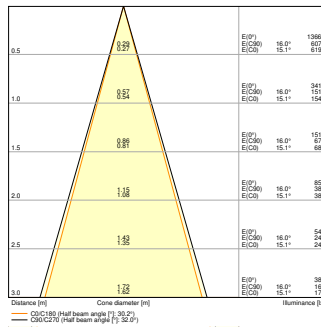
UB WL VARIO RD 29W ML 830 GY 30D Up Down
