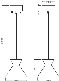
DECOR WAIST PENDANT E27
