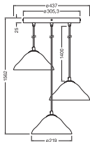
DECOR LOTUS LEAF PENDANT 3XE14 WT
