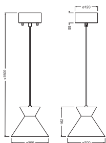
DECOR WAIST PENDANT E27
