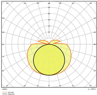
LDVAL BAT HE 900 9.6W G3 24X1 EN LEDV
