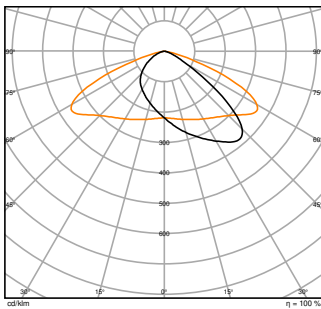
FL PFM DA 290W 4000K ASYM 45X140 BK
