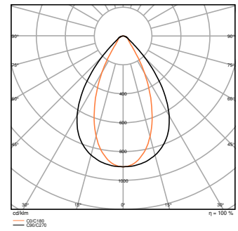
LB FLEX 1500 P 140W 840 OV
