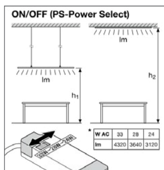
PL CMFT 1200 33W/840 UGR19 PS Lichtstroomelectie met Multi Lumen switch (CRI80 versies)
