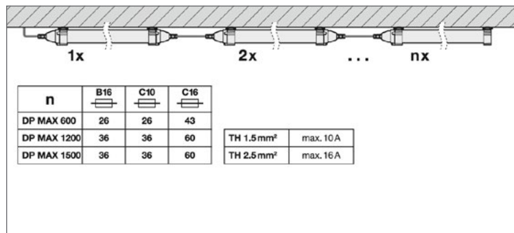
DP MAX - Aantal per installatie-automaat
