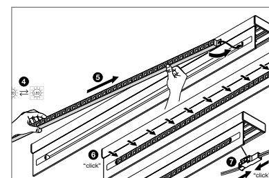
Vervanging van de lichtbron
