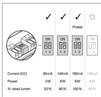
Instellen van de microschakelaars
