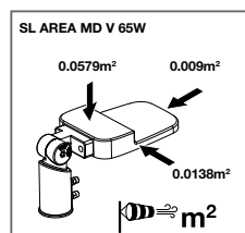
Invloed wind
