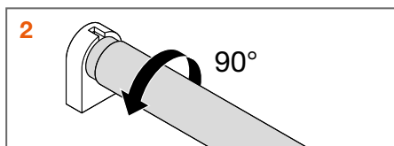
T8-Röhre entriegeln.
