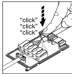
Werkzeuglose Anschlussklemme und Zugentlastung
