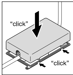
Werkzeugloses Öffnen und Schließen der Anschlussdose
