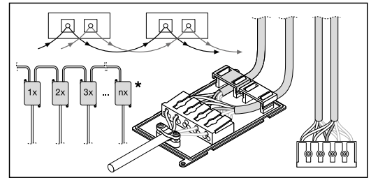
Mitgelieferte 5-polige Klemme ermöglicht Durchgangsverdrahtung
